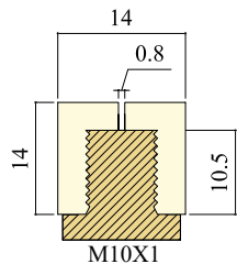
Art. 7345 FERRULE JBR "S2-S3-S5-S20" CAROM - 5 SKITTLES - WOOD - PRO SERIE (PRO, PRO2, PRO3, PRO4) GHIERA JBR "S2-S3-S5-S20" CARAMBOLA - 5 BIRILLI - LEGNO - SERIE PRO (PRO, PRO2, PRO3, PRO4)
