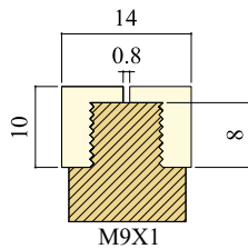
Art. 7345 FERRULE JBR "S2-S3-S5-S20" CAROM - 5 SKITTLES - WOOD - PRO SERIE (PRO, PRO2, PRO3, PRO4) GHIERA JBR "S2-S3-S5-S20" CARAMBOLA - 5 BIRILLI - LEGNO - SERIE PRO (PRO, PRO2, PRO3, PRO4)
