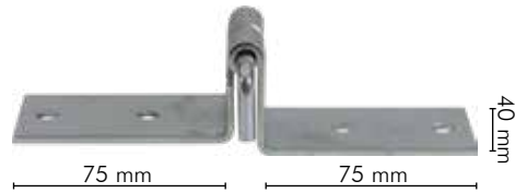
Art. 300265 Hinge for soccertables mod. Longoni Cerniera per calcetto serie Longoni
