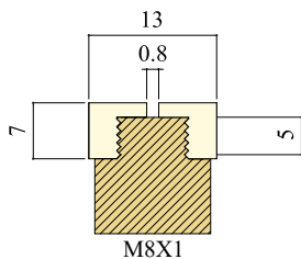
Art. 7345 FERRULE JBR "S2-S3-S5-S20" CAROM - 5 SKITTLES - WOOD - PRO SERIE (PRO, PRO2, PRO3, PRO4) GHIERA JBR "S2-S3-S5-S20" CARAMBOLA - 5 BIRILLI - LEGNO - SERIE PRO (PRO, PRO2, PRO3, PRO4)
