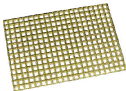
ART. 302118O COMPACT PROTECTION GRID (305 X 205 X 8 mm) GRIGLIA ORO PER LAMPADARIO COMPACT (305 X 205 X 8 mm)
