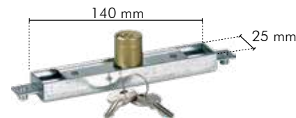
Art. 300185 Lock for soccer table Serratura per calcetto
