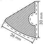
art. 7079 Rubber cushion n°66 BIBA ROT 6 pcs set for 9' pool table (Set price) Gomma n°66 BIBA ROT set 6 pz. per pool 9' (Prezzo per set)
